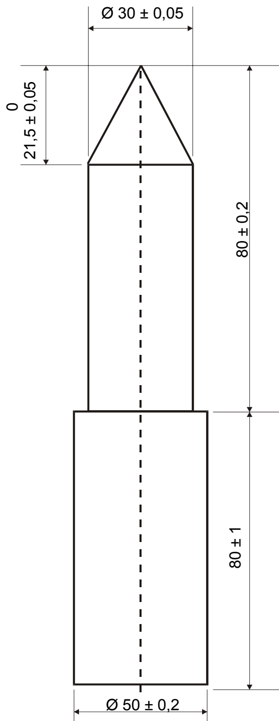
Figura 4. Probeta de prueba
