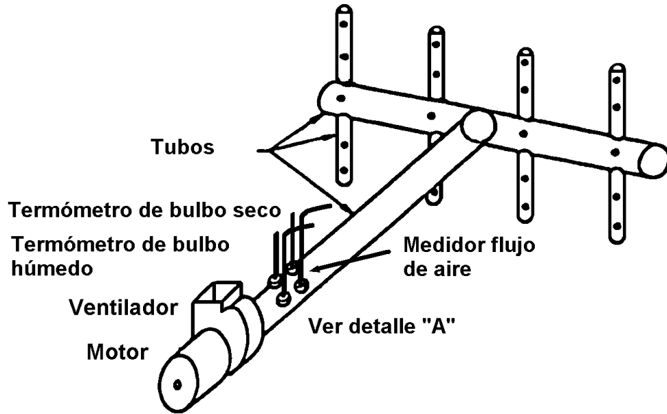
Figura C.1 Dispositivo de toma de muestra de aire para la unidad de prueba o el equipo de acondicionamiento.
