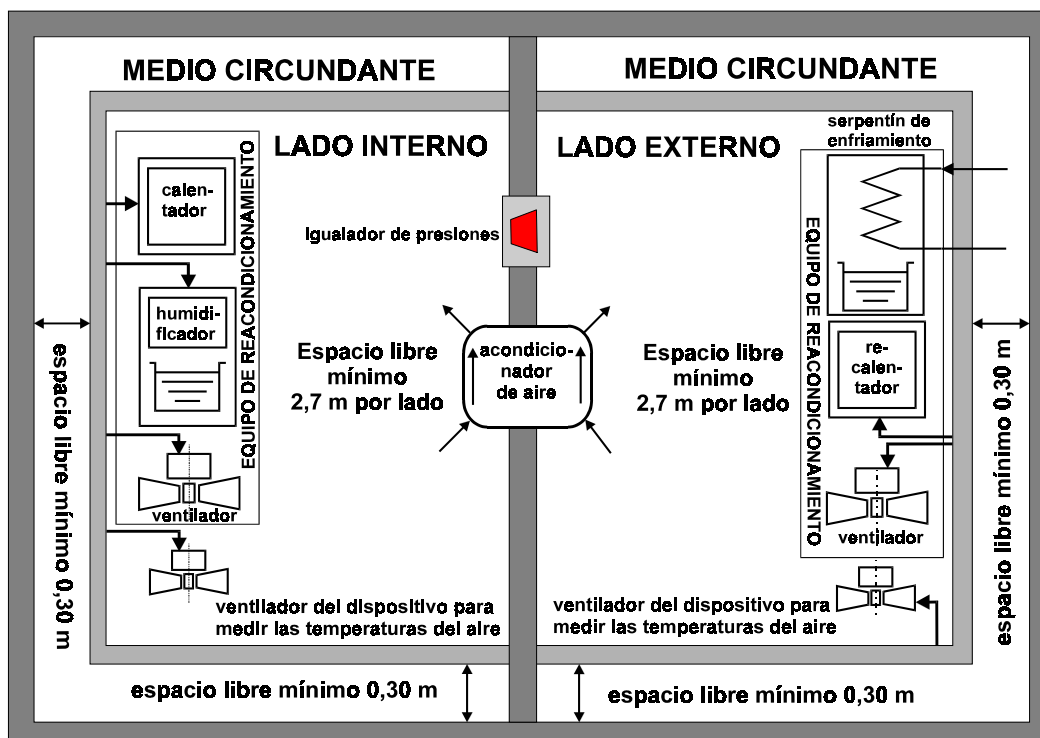
Figura 1. Calorímetro de cuarto tipo ambiente balanceado
