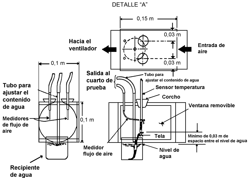
Figura C.2 Dispositivo para toma de temperatura de bulbo húmedo
