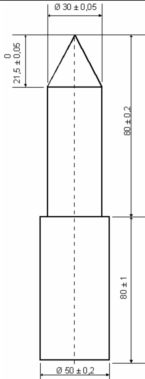
Figura 4. Probeta de prueba
