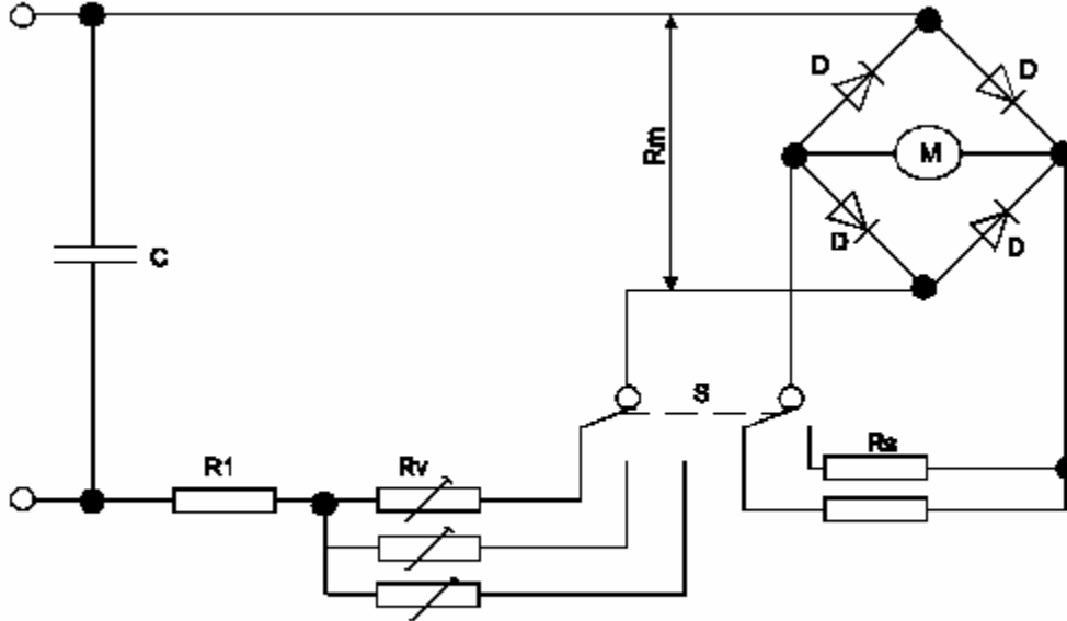
Figura 1 Circuito para medir corriente de fuga
